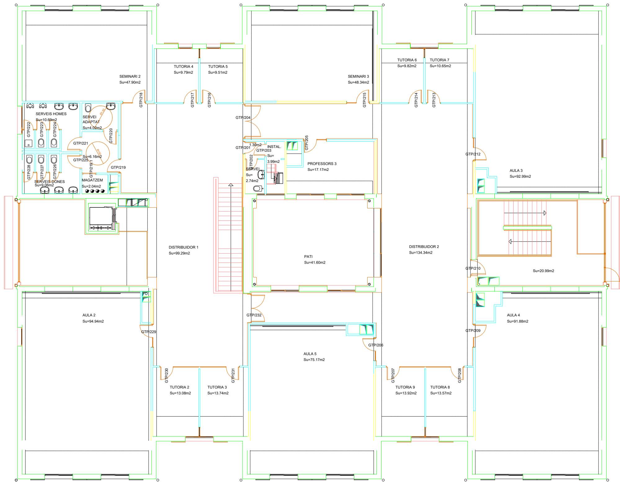
PLANTA SEGONA
